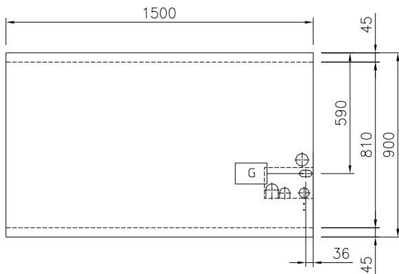
Boven aanzicht
